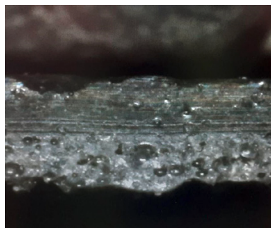
Querschnitt einer Slush-Haut: Damit der Airbag sicher auslöst, muss die Sollrisstelle bis in die oberste Schicht eingebracht werden.
